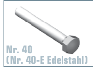
Schraube M8 gem. DIN 558, Länge (mm): 30, 40, 60, 80, 100 und 120
