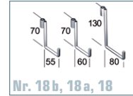
Hakenbefestigung Nr. 18 130 x 80 mm Nr. 18a 70 x 60 mm Nr. 18b 70 x 55 mm
